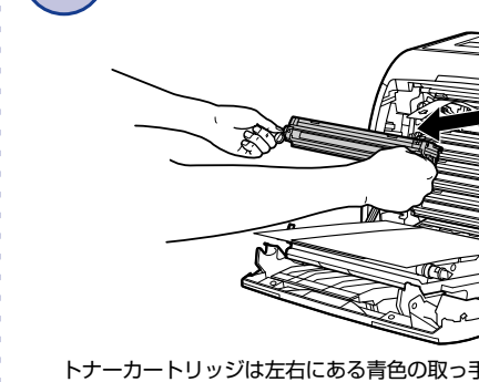
トナーカートリッジは左右にある青色の取っ手を持ち、水平に引き抜きます。トナーカートリッジはしっかりと両手で持って、ETBユニットの搬送ベルトに当たらないように引き抜きます。
