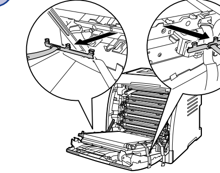
梱包材は、垂直方向ではなく、プリンタ斜めに取り外します。
