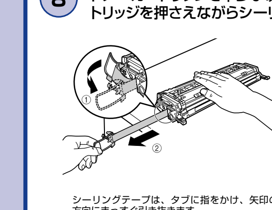
シーリングテープは、タブに指をかけ、矢印の方向にまっすぐ引き抜きます。
